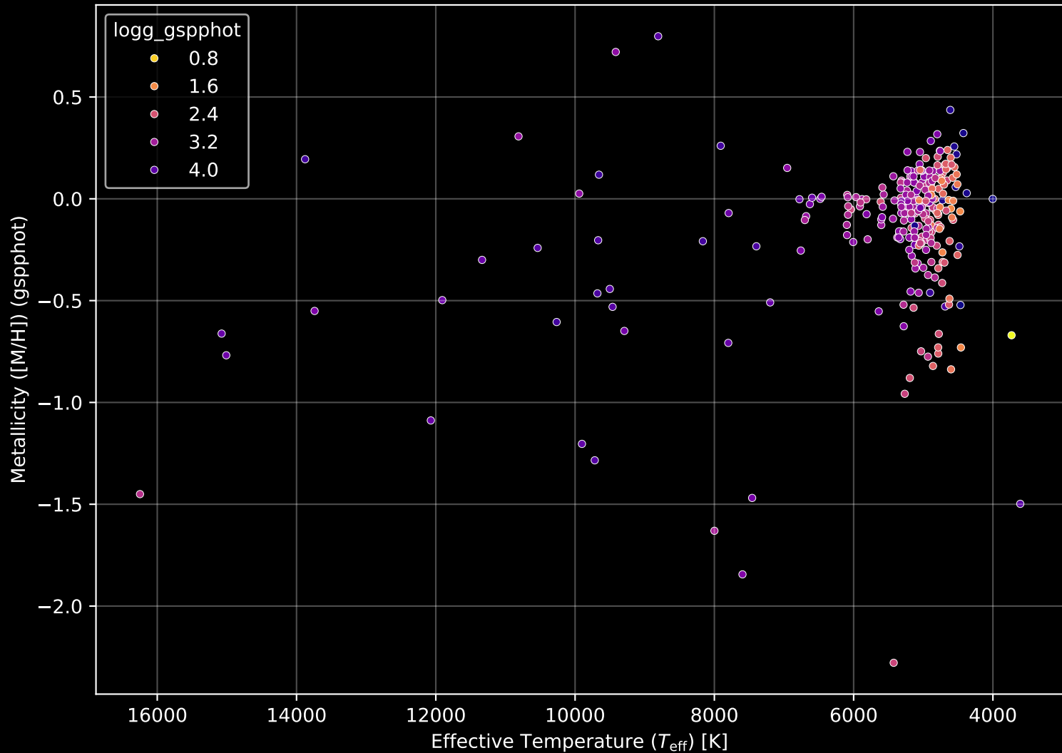
APOGEE DR17 Field: [109+08] Stellar Population Parameters (n= 278)
